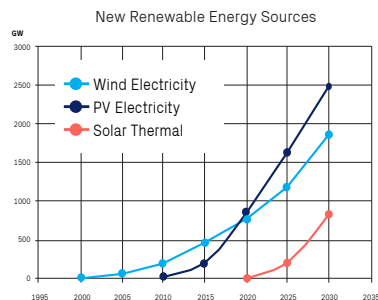
Illustration av tillväxt hos vind, solceller och en kommande tillväxt för solvärme inom industrin från dagens nivå om någon GWth till 850 GWth år 2030
